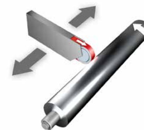
Retificação cilíndrica de bielas de pistões e cilindros, p. ex. entre pontas
